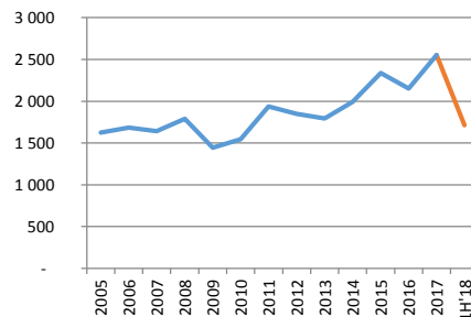
Średnia dyspozycyjność* mocy z wiatru w Polsce [godz./rok]
